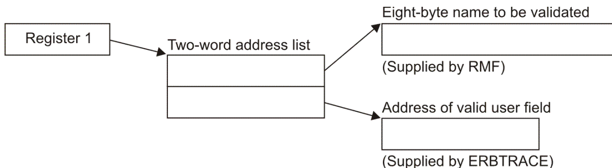
Figure 14. ERBTRACE Input Parameter Structure
