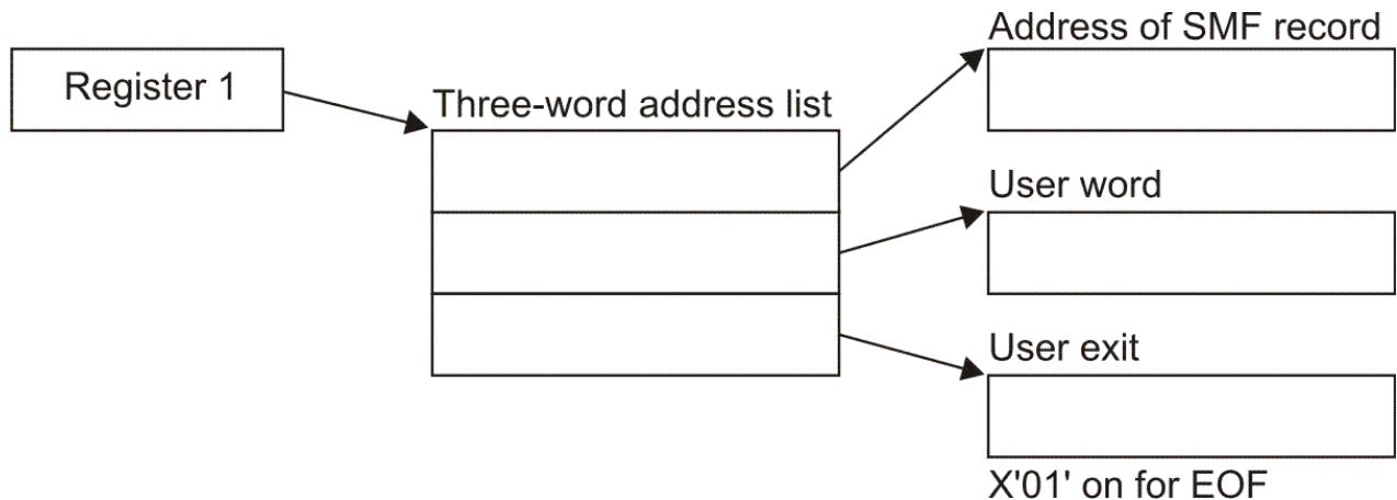
Figure 15. ERBMFPUS Input Parameter Structure
