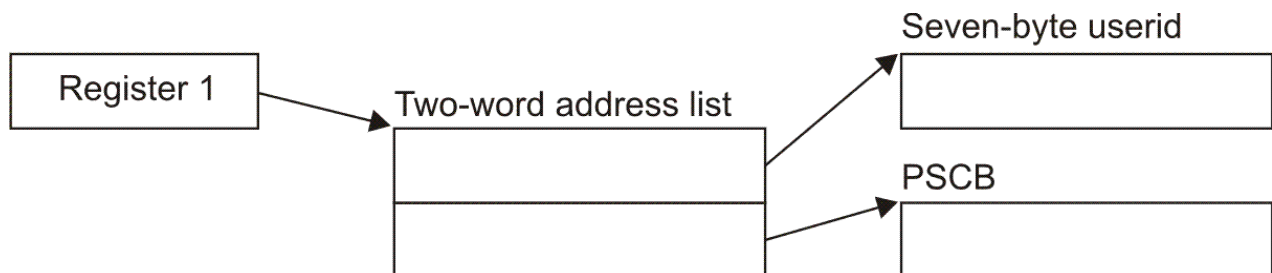
Figure 22. ERBTSOCK Input Parameter Structure
